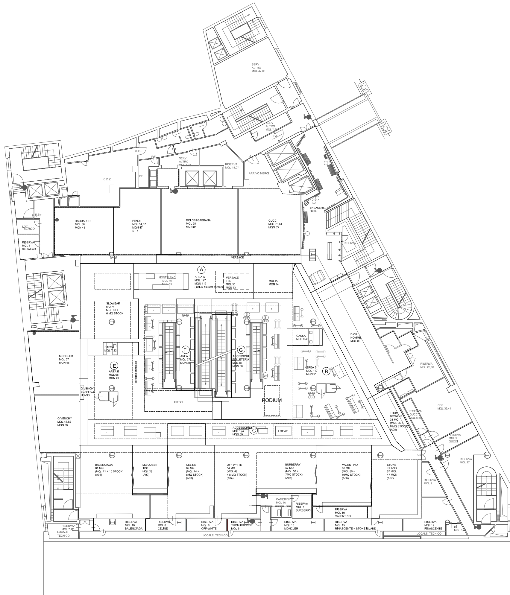
LAYOUT GENERALE PIANO PRIMO_MILANO
